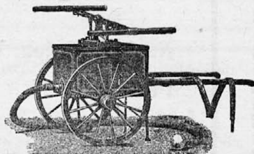
Dvokolna brizgalnica, podvojeno brizgajoča 180 — 200 2 /min.
