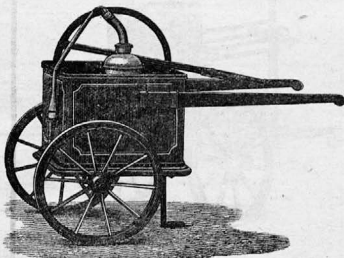
Dvokolna brizgalnica, pripravna za gospodarske in tovarniške zavode.
