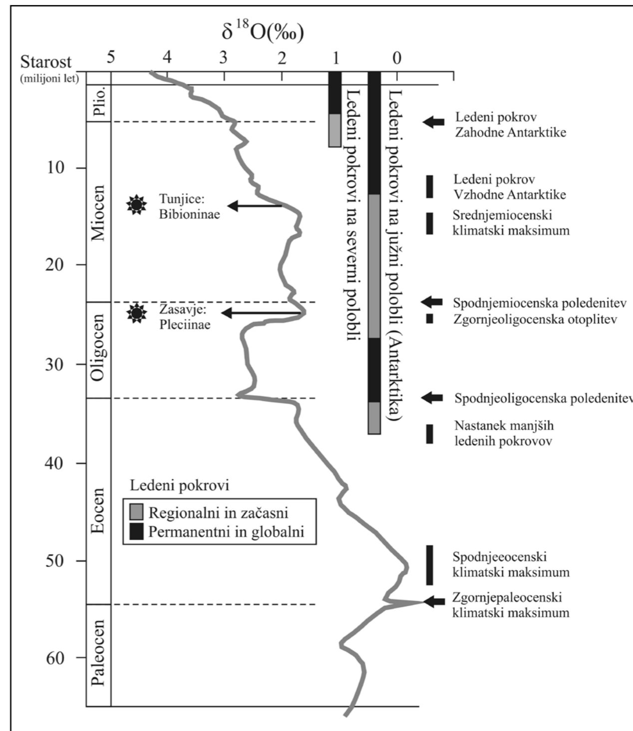
Slika 7: Evolucija kenozojske globalne krivulje deleža izotopa 180 (‰) v morskem okolju (prilagojeno po Zachos et al., 2001), ki kaže tendenco temperaturnih variacij.
