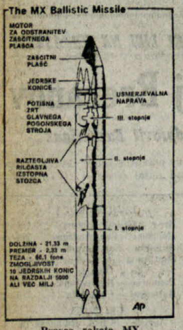
Prerez rakete MX
