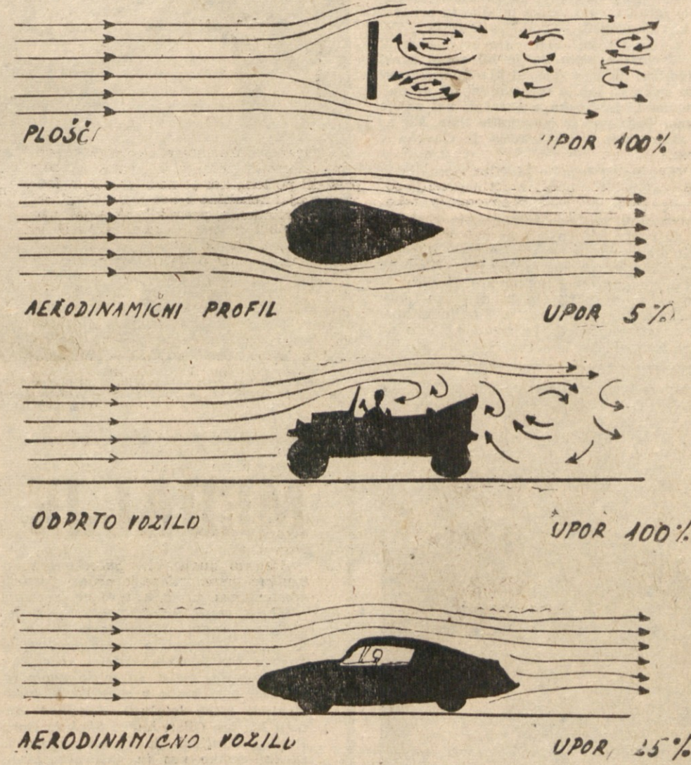
Nekaj primerjav teles v zračnem toku. Stari avtomobili se zelo približujejo uporu, ki ga ima ravna plošča in so bili zato kljub razmeroma močnim motorjem zelo počasni
