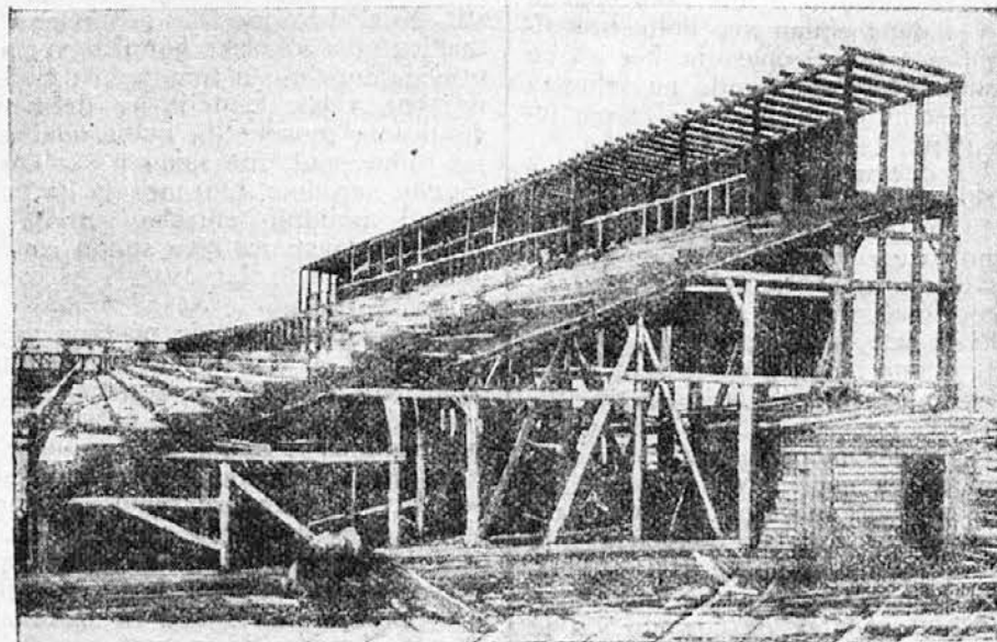
Slika prikazuje prosek glavne zapadne tribine za vreme gradnje. To je samo jedna polovica zapadne tribine, koja je svega 233 metra duga. U sredini je posebna loža Nj. Vel. Kralja, Visokog Pokrovitelja zagrebačkog sokolskog sleta. Gore u visini od 10 metara su lože, pred njima na stepenicama sedišta, a dole pred sedištima (na slici se ne vide) stepenice stajališta. Na zapadnoj tribini biće mesta za sedenje za 7000 gledalaca.
