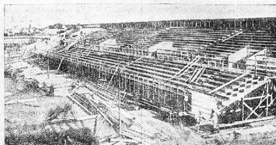
Pogled na severnu tribinu velikog sokolskog sletišta u Zagrebu. Isto takva je i južna tribina. Obe zatvaraju vežbalište s kraće strane, a duge su svaka 177,05 metara, široke 19,10 metara, a visoke 9,70. Na tim »kraćim« tribinama biće mesta za 5200 sedišta, na svakoj. Svega, na svim tribinama sletišta ima 23.000 sedišta, a u stajalištu mesta za 30.000 ljudi. Dakle svega za 53.000 gledalaca, a može da stane još više.
