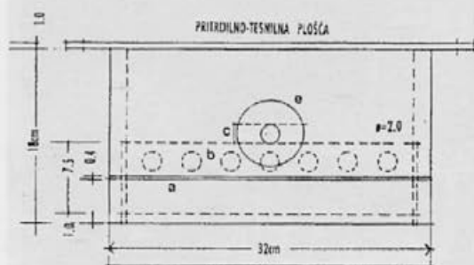
TLORIS
