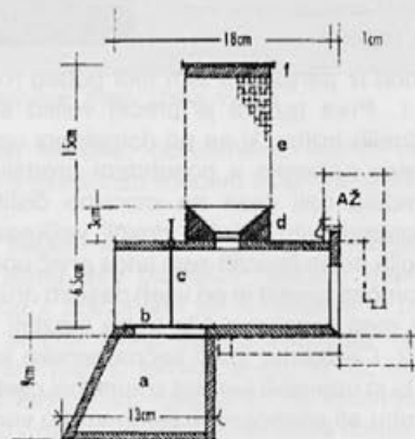
PREČNI PREREZ
