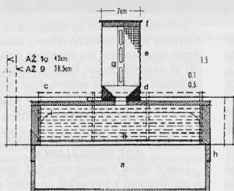
VZDOLŽNI PREREZ
