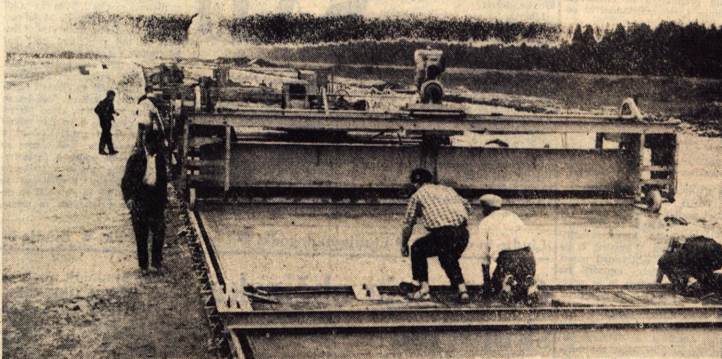
Dela pri gradnji modernega letališča v Brnikih hitro napredujejo ob uporabi vse sodobne mehanizacije, ki jo ima na razpolago gradbeno podjetje Slovenija-cesta
