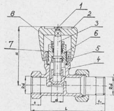
Radiatorski ventil
