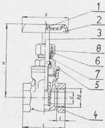
Zaporni zasun
