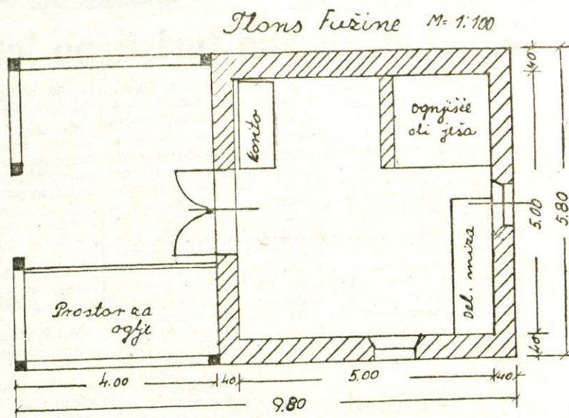
Tloris fužine, v kateri izdelujejo zvonce; merilo 1:100
