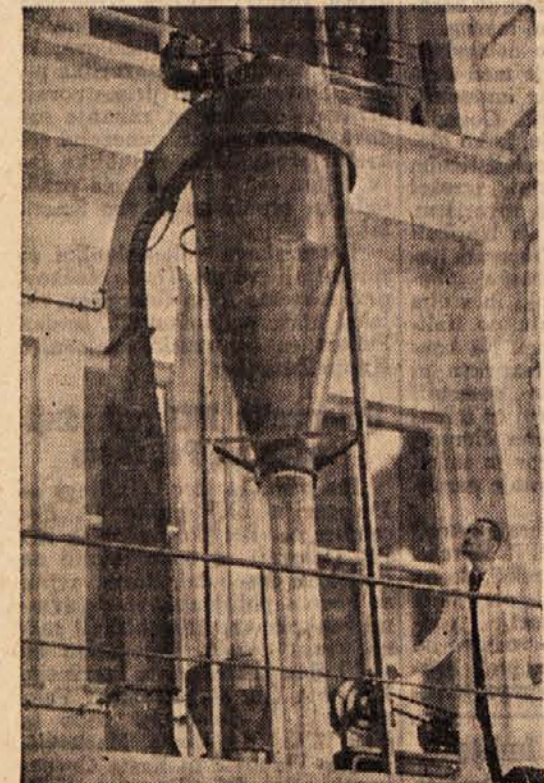
Aparat za klasifikacijo azbesta je najnovejša pridobitev Zavoda za proučevanje gradbenega materiala
