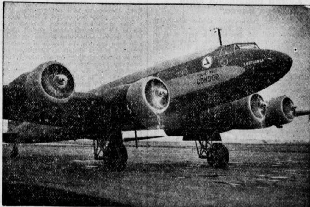
Prvikrat v zgodovini je letelo letalo tipa Focke-Wulf-Condor naravnost iz Berlina v Ameriko, ne da bi kaj pristalo spotoma in je že čez 25 ur srečno prispelo v New York. Proga meri 6500 kilometrov, bencina je letalo porabilo 9000 litrov. Svetovno časopisje živahno razpravlja o tem uspehu nemškega letalstva.
