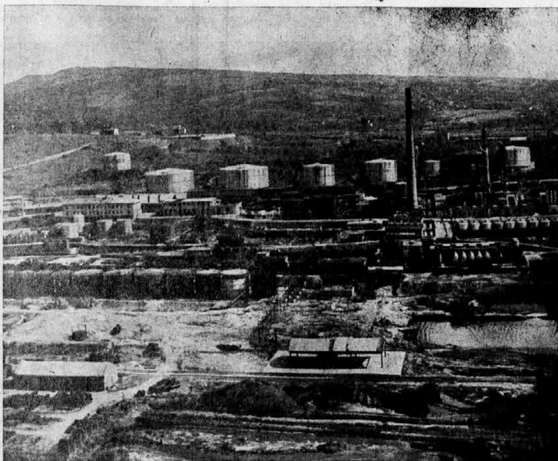
Tržaška petrolejska rafinerija »Aquila«, ki so jo na novo zgradili s pomočjo sredstev Marshallova načrta, bo kmalu ena najmodernejših v Evropi.
