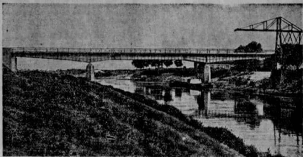
Železen most brez zakovice. Most je dolg 80 m; posamezni deli so med seboj zvarjeni in ni na vsem mostu niti ene zakovice. To je prvi most te vrste v Nemčiji. Most veže oba bregova reke Aller pri Verdenu
