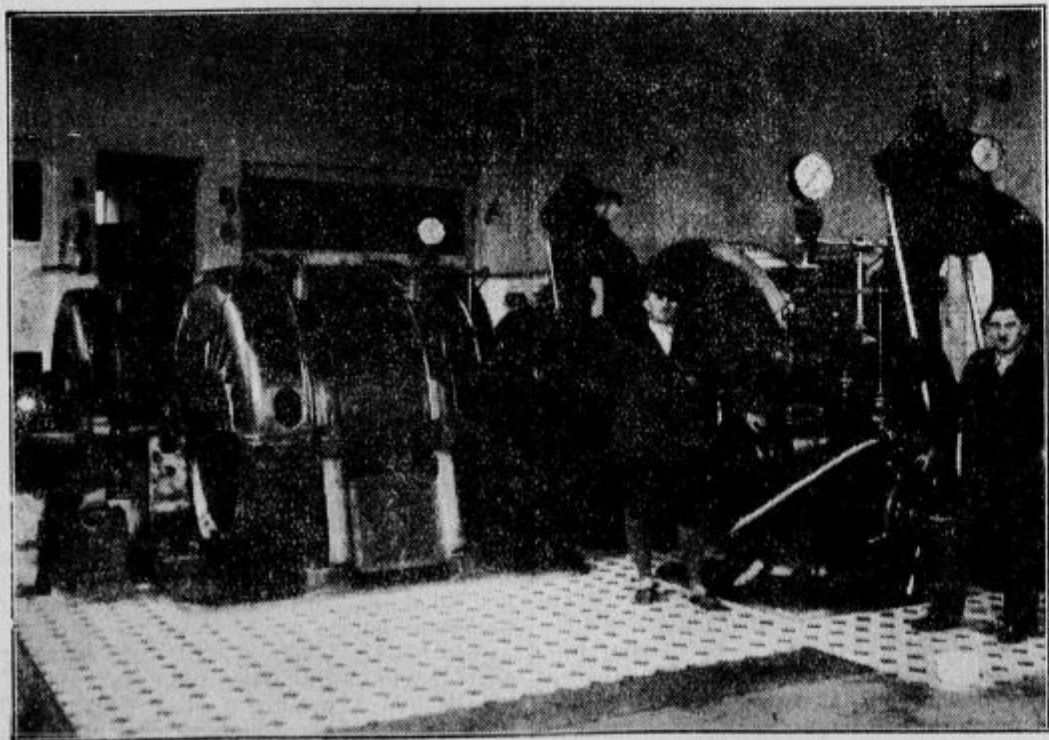
Stroji v elektrarni grmijo. Od leve na desno: generator, vztrajnik z regulatorjem ter turbina. Zač: se vidi druga garnitura strojev, ki počiva.
