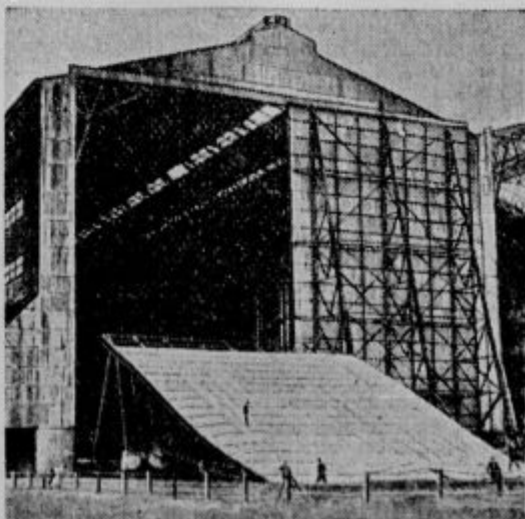
Po strahoviti katastrofi, ki je doletela angleški zrakoplov »R. 101«, je Anglija sklenila opustiti zrakoplove. Na sliki razdirajo zrakoplovno lopo v Howdenu. Pravkar so sneli vrata, ki so bila 70 m visoka, in so tehtala 200 ton.
