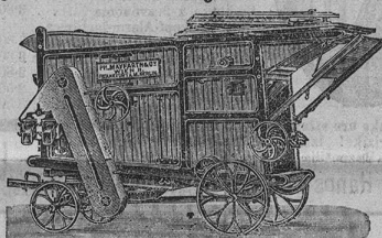
Mašine za mlaiti s patent Rolch-Ringschmeller za prorit na roko, motor ili gopel
