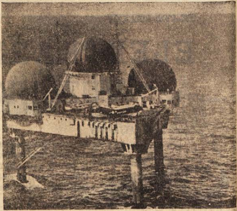
Oporišče sredi Atlantika. Vojaško poveljstvo ZDA gradi več oporišč, ki so približno 100 do 120 milj oddaljena od obale. To so dejansko radarske opazovalnice. Njihova glavna naloga je, da se pravočasno opozorijo na morebiten napad sovražnih letalskih sil. Oporišče je postavljeno na treh plavajočih stebrih, v treh kupolah pa so radarske opazovalnice. Na ploščadi, ki jo vidite v ospredju slike, pa pristajajo helikopterji, ki vzdržujejo zvezo med oporiščem in celino.
