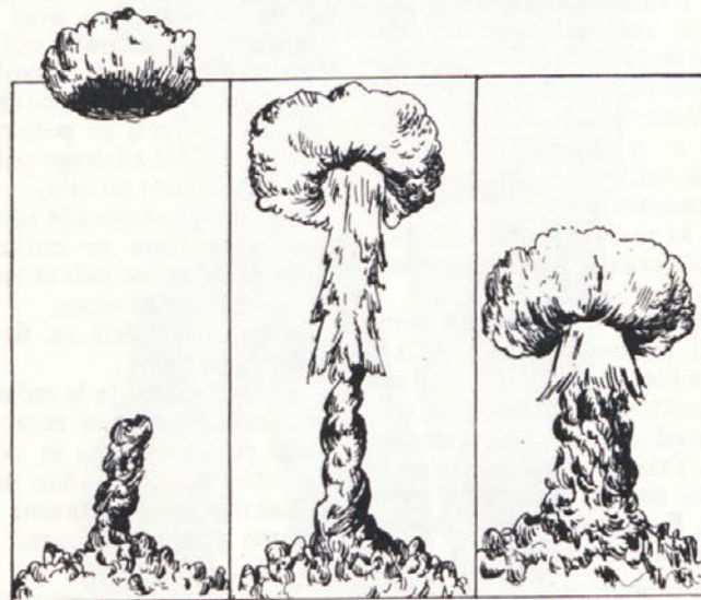
Sl. 9. Videz atomske gobe: A. pri eksploziji višje v ozračju, B. pri eksploziji nižje v ozračju, C. pri površinski eksploziji
