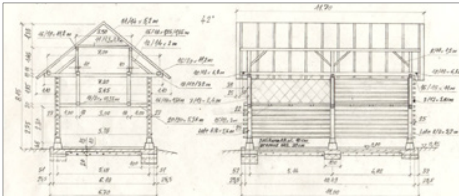
Izris kozolca toplarja s štirimi štanti
