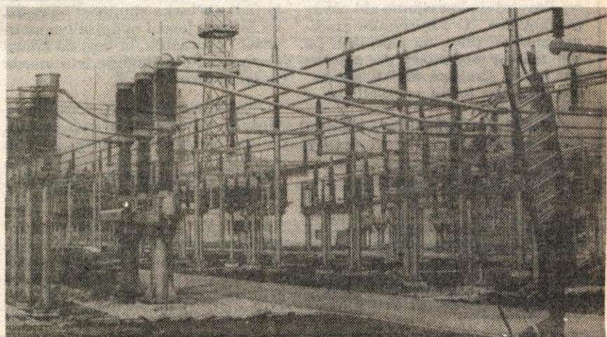
Razdelilna transformatorska postaja Okroglo pri Kranju bo vzliščje elektroenergetskih zvez na Gorenjskem. Z njo bo rešeno kritično napajanje Gorenjske z elektriko, pomembna pa je za napajanje nove elektroeklarne na Jesenicah. Graditi so jo začeli junija leta 1982, vse kaže, da bo kon-
