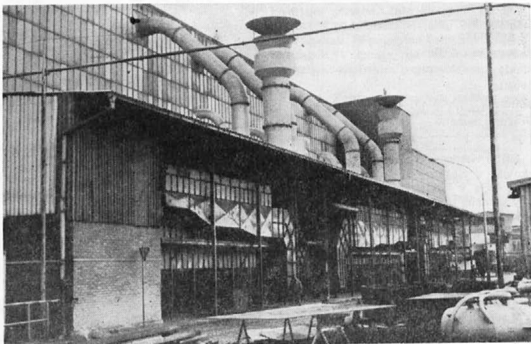
»Opešana« italijanska odpraševalna naprava pri novi jeklarni
