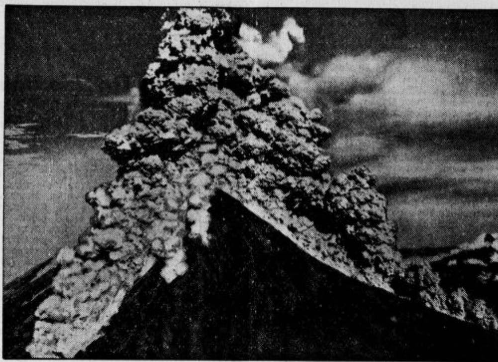
Ognjenik Mayon na Filipinih je meseca junija začel bruhati. Kamenje in lavo je metalo več sto metrov visoko. Slika je iz večje daljave posnelo ameriško vojno letalo
