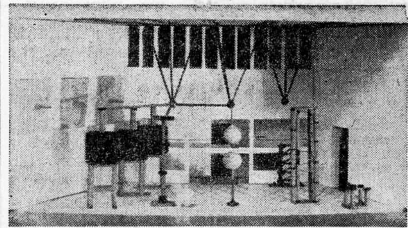
Model laboratorija za visoko napetost, v katerem bodo naši strokovnjaki preizkušali izolacijske snovi in električne naprave z napetostjo do 2 milijona voltov.
