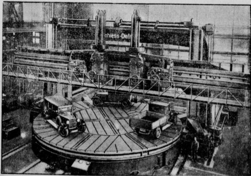
Največja stružnica na svetu. Orjaška vrtiljačasta stružnica, ki ima premer 22,5 metrov in tehta 1400 ton. Služi za obdelavo turbinskih ležajev.
