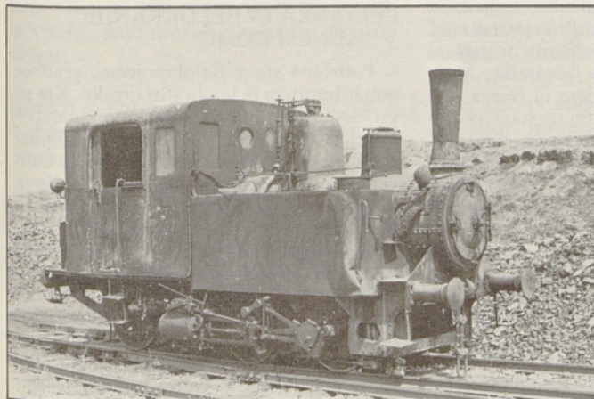
Lokomotiva JDŽ 162 ima pogonske cilindre zadaj in je kot taka izredna tehniška posebnost.
