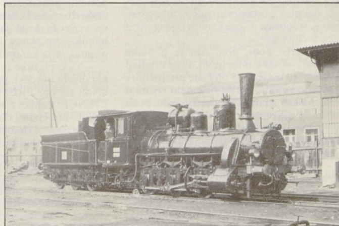
Lokomotiva JDŽ 125 z nizkoležečim kotlom in zunanjim nosilnim okvirjem.
