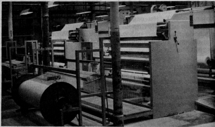
S prestavitvijo Malipol in Schusspol strojev v staro tkalnico, tako da se je formiral zaključen oddelek pletilnice, smo pridobili prostor za postavitev Terhaerst tkalskega stroja.
