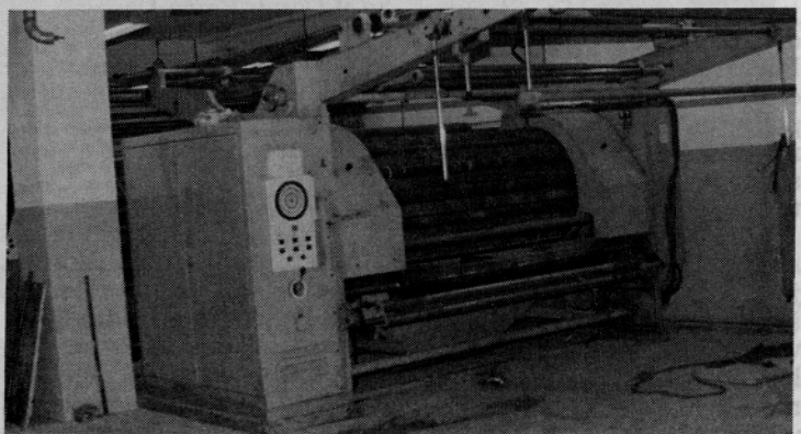
V bivšo sukalnico prestavljeni kosmatilni stroji — sprostitev prostora za postavitev nove investicijske opreme v Oplemenitilnici.
