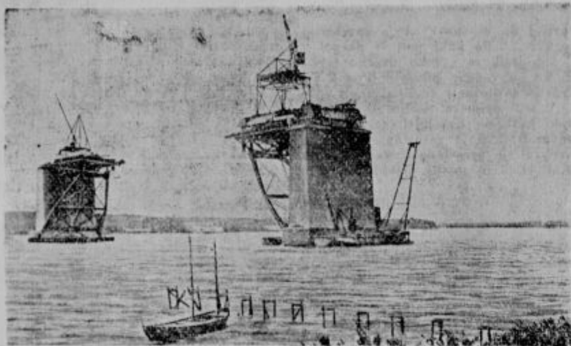
Najdaljši most v Evropi postavljajo Danci čez Mali Belt. Na sliki vidimo dva stranska stebra bodočega mostu, med katerima se razvija parniški promet. Stebra se dvigata 30 metrov visoko nad morsk gladino.
