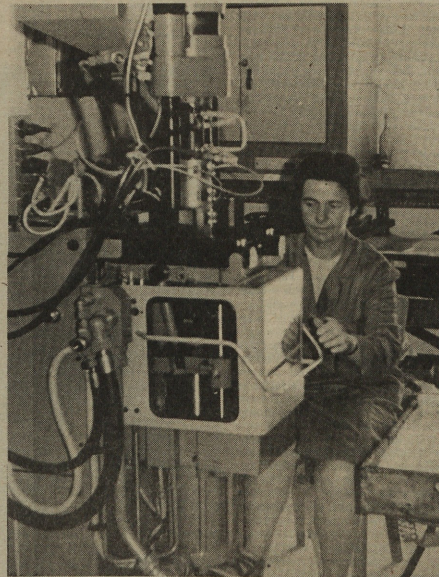
Zaradi premajhnih strojnih kapacitet se je vodstvo Tovarne električnih merilnih instrumentov v Otočah odločilo za nakup modernih strojev za brizganje plastičnih mas, avtomatov in polavtomatov za obdelavo kovinskih delov ter za orodjarno. Na sliki Francka Frelj pri novem, modernem stroju za brizganje plastičnih mas.
