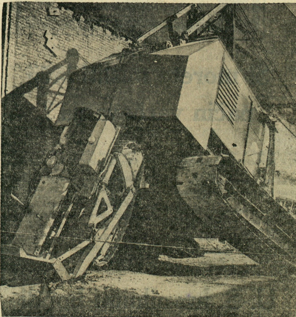
SPOPAD BULDOZARJEV? -- Nekaj takega se je dogodilo lani v bližini Clevelanda, ko sta se sprla voznila dveh buldozerjev različne velikosti, vole na sliki pa je nastalo po nesreči, to se je zlomila ruka velikega žerjava s premalo težo vozila. Mali buldozer je pomagal držati vozilo žerjava k tlom. To je bilo še vedno prelahko in se je dvignilo od tal. Ko se je roka žerjava zlomila, je "hišica" žerjava običajna na buldozerju.
