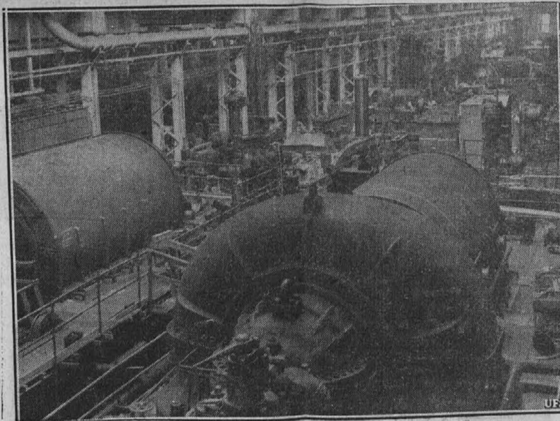
Ogromno kolesje za narodno obrambo. — Delavci v General Electric tovarni v Schenectady, N. Y. so zaposleni 24 ur na dan, da lahko izgotovijo naročila za turbine, ki se jih rabi pri narodni obrambi. Tovarna ima v delu 3 turbine, katerih vsaka bo proizvajala 60,000 kilovatnih ur elektrike.
