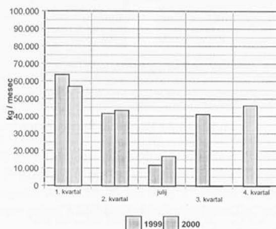
Pregled distribucije hladilne vode za leto 1999 in 2000
