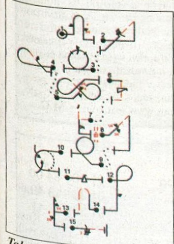
Tako izgleda načrt programa akrobacij, ki ga ima pilot ob instrumentih pred sabo.
