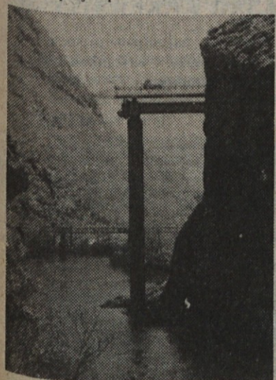
Podporni steber, ki je visok skoraj 70 metrov, bo nato, ko se bo napolnilo akumulacijsko jezero HE Višegrad le nekaj metrov nad vodno gladino.
