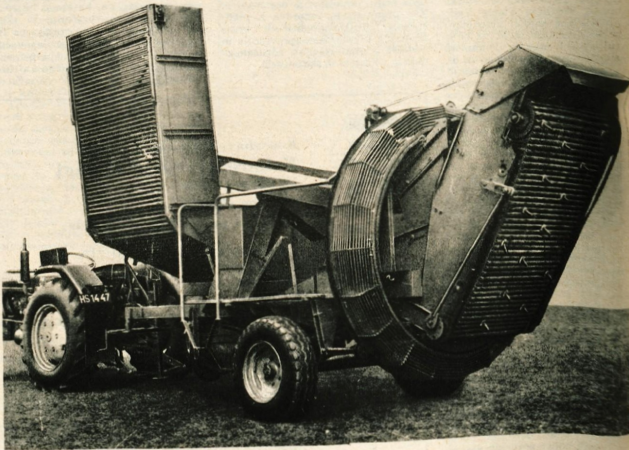
Kombajn za izkopavanje krompirja po licenci WÜHLMAUS
