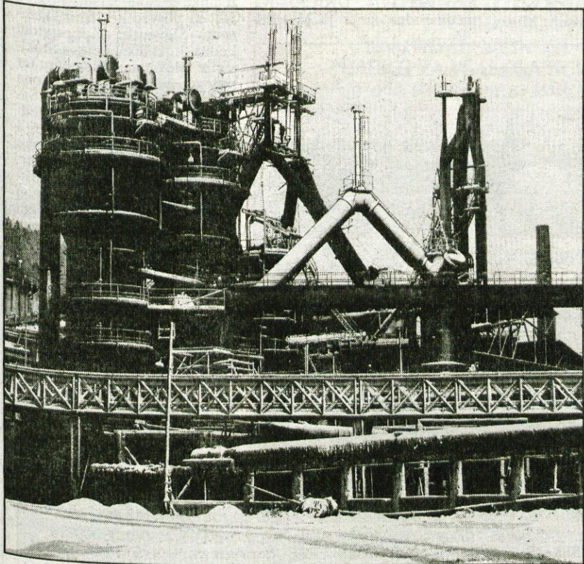
Zimski posnetek stolpnih plinskih čistilcev s plavžema
