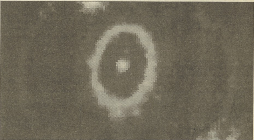
Allan Sandage si pri ugotavljanju starosti vesolja pomaga s svetlobo supernove.
