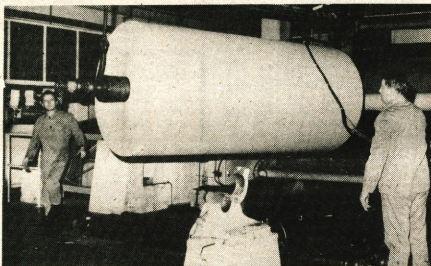
Papirni stroj v tržiški Lepenki obratuje noč in dan. Streže mu pet ljudi. Ustavi se le štirikrat na leto. — Foto: F. Perdan
