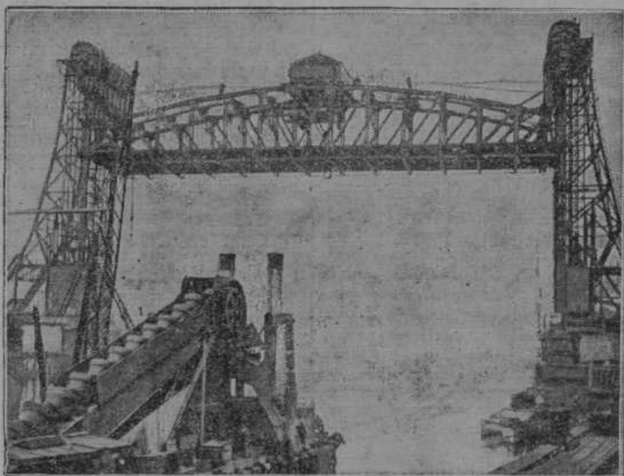
Prvi most, ki se da dvigniti, so dogotovili pri Newportu preko reke Tees na Angleškem. Most je širok 18 m, prostor za vozila 11.60 m in oba hodnika za pešce vsak po 2.75 m. Stolpa ob straneh sta visoka 47.7 m in znaša dvigalna višina 36.5 m.
