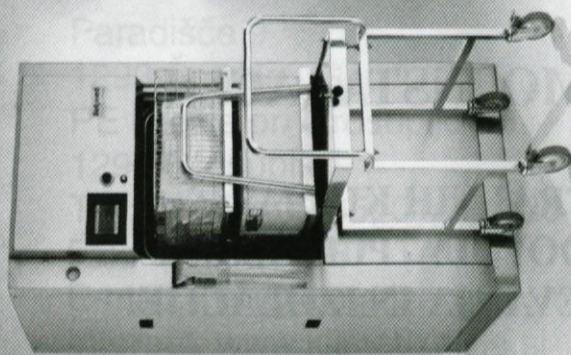
Medicinski parni sterilizator tip MST-V
