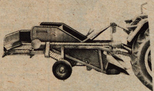
Niewöhner-wühlmaus IZKOPALNIK KROMPIRJA z verižno pretresalno napravo v domači in uvoženi izvedbi.
