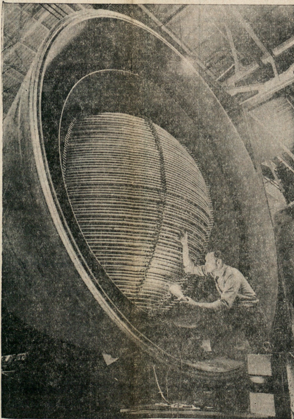
PARNI GENERATOR — Slika kaže tehnika Westinghouse družbe pri pregledu odprte cevi velikega parnega generatorja, ki bo nameščen v atomski elektrarni pri Buchananu, N.Y. V generatorju je 39 milj cevi.
