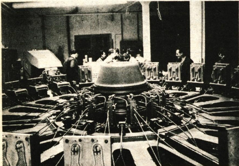
Moderni stroji že leta in leta pomagajo pri uveljavljanju Peka doma in na tujem. Na fotografiji moderen stroj za vlijanje poliuretanskih podplatov Desma
