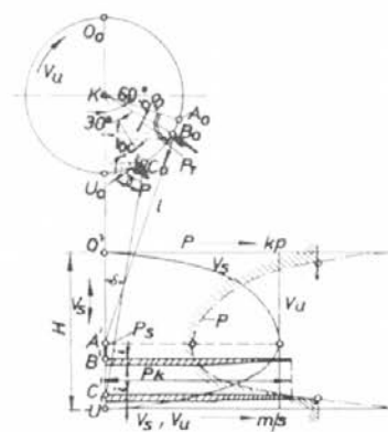
Slika 2 — razpoložljiva sila stiskalnice P in rezalna sila P_k . Rezalna sila mora biti manjša od razpoložljive sile stiskalnice.
