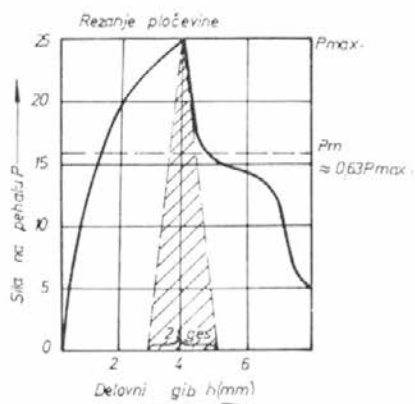
Slika 1 — potek sile rezanja v odvisnosti od kota zasuka ročične gredi ali hoda pehala
