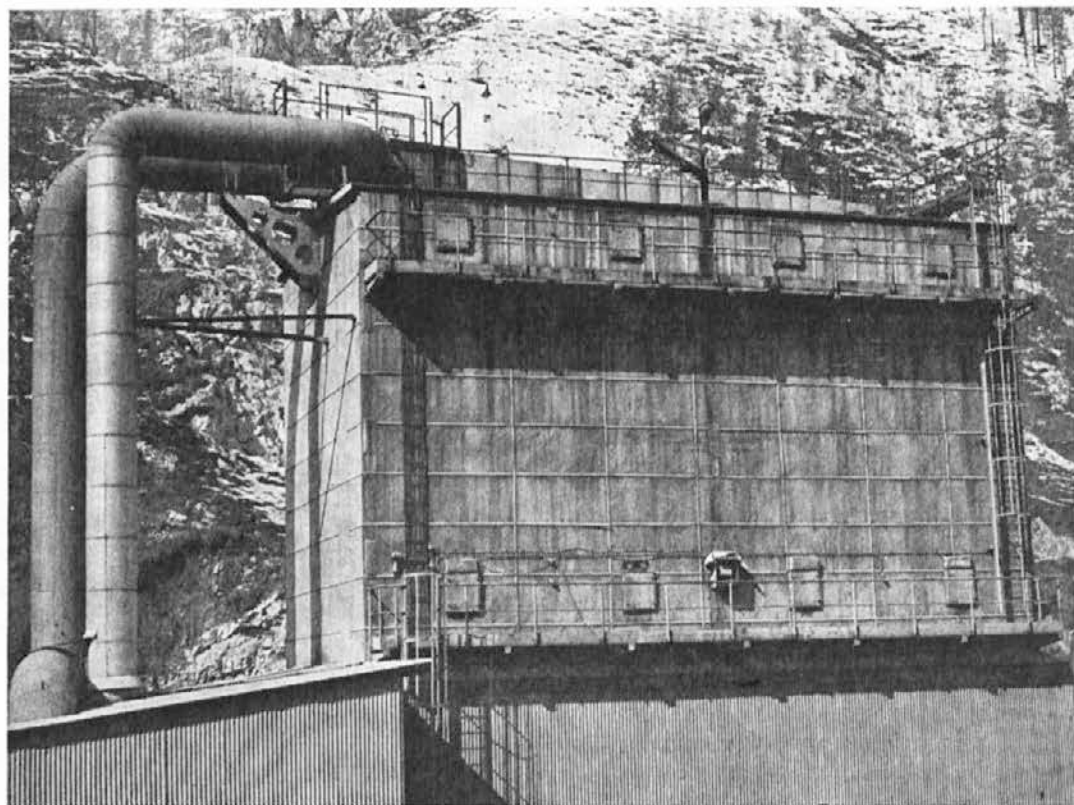
»Novi lurgi«, obratuje od leta 1968
