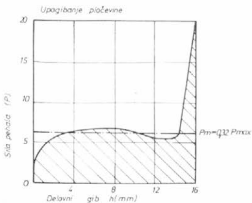
Slika 4 — potek preoblikovalne sile pri upogibanju
