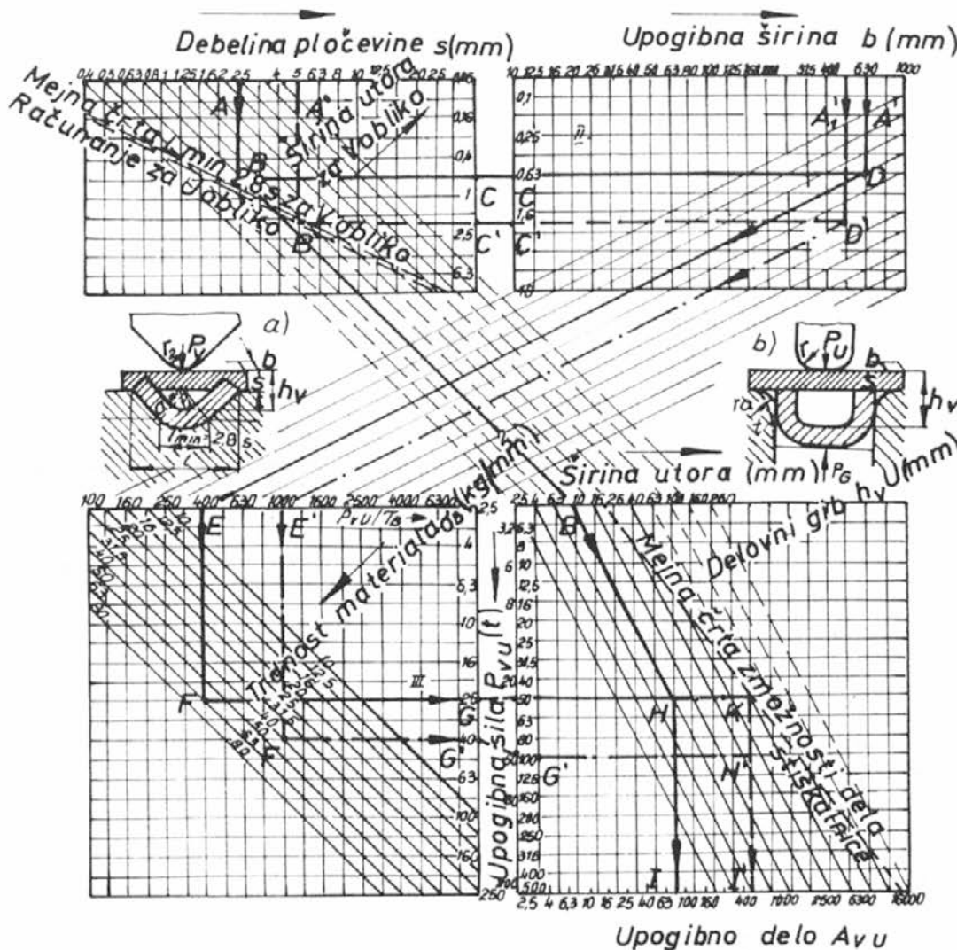
Slika 5 — diagram določanja upogibne sile in dela, potrebnega za upogibanje
