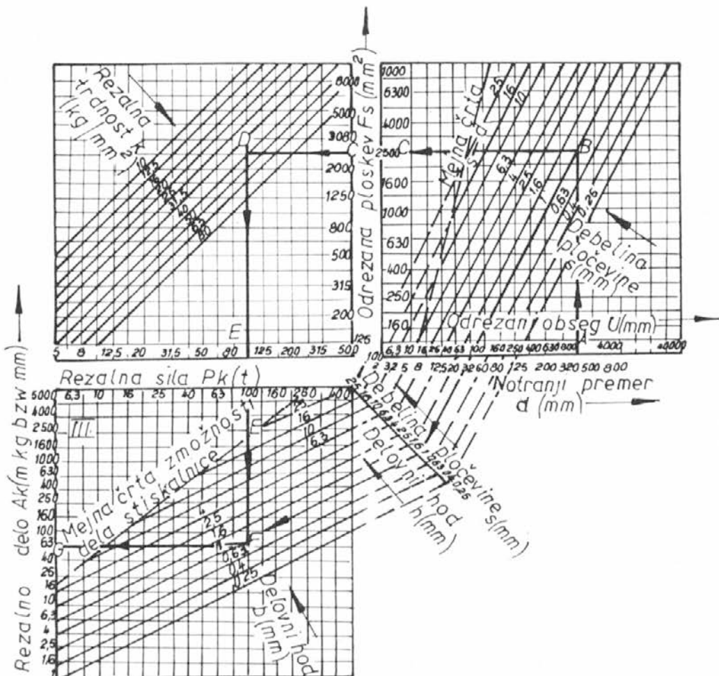
Slika 3 — diagram določevanja rezalne sile in potrebnega dela za rezanje
