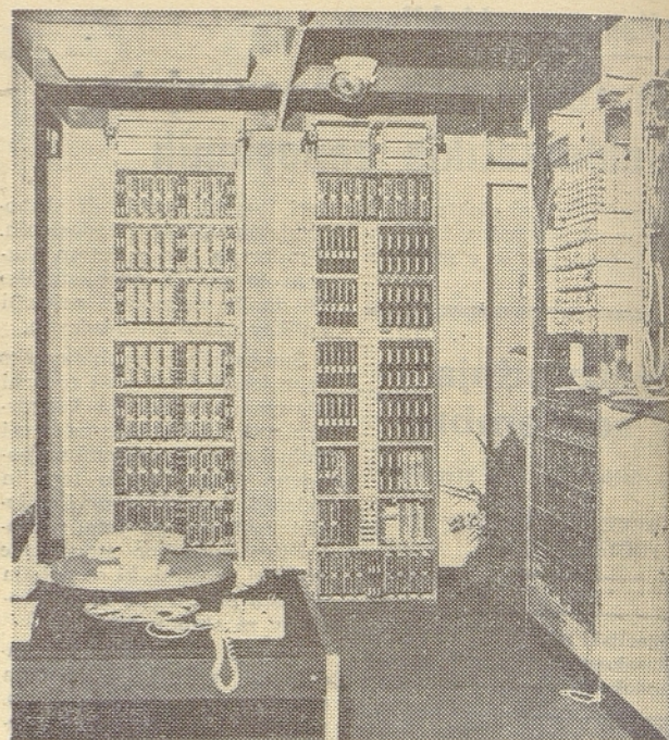
Takšna je videti telefonska centrala Metaconta 10 C, ki jih bo Iskra dobavila vrsti naših ptt podjetij, ki si prizadevajo modernizirati telefonski promet pri nas
