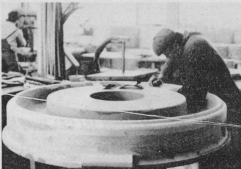
Posnetek iz modelarne. Pred lakiranjem je treba model pokitati in izbrusiti.
