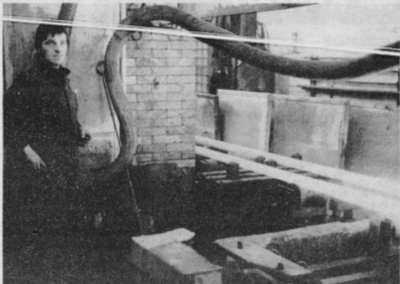
Posnetek iz livarne, kjer vidimo dvožilno vlečenje kontinuirane sive litine.
