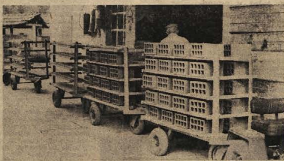
Polizdelki — surova opeka — čakajo, da jih bodo izpred strojnice odpeljali v sušilnico. Zdaj ta prevoz brez človeka ne gre, prihodnje leto pa bodo prevoz upravljali že elektronsko s komandne plošče
