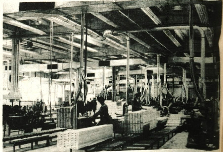
Zaradi sodobne opreme je bilo potrebno na eni izmeni zaposliti le 30 delavcev — Foto: F. Perdan
