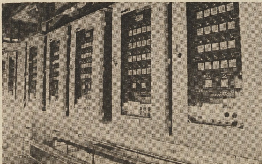
Že v prejšnji številki smo poročali, da je bila v TOZD SVN izdelana 3.000. centrala za javljanje požara.
