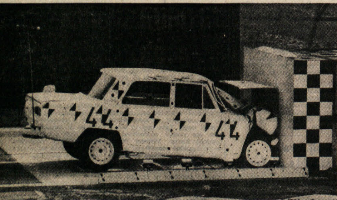
«Berlina 1700» znamke «alfa - romeo» po poskusu, ki so ga izvršili na avtomobilski progi Balocco. Avto je trčil v cementni zid s hitrostjo 50 km na uro. Pri tem se je prednji del hudo pokvaril, vozniški prostor je pa ostal nepoškodovan. Izvedenci skušajo doseči, da bi pločevina delovala pri trčenju kot «blazina» in omiliha sunek. Veliko pažnje polagajo izvedenci tudi volanu in bencinskemu rezervoarju.
