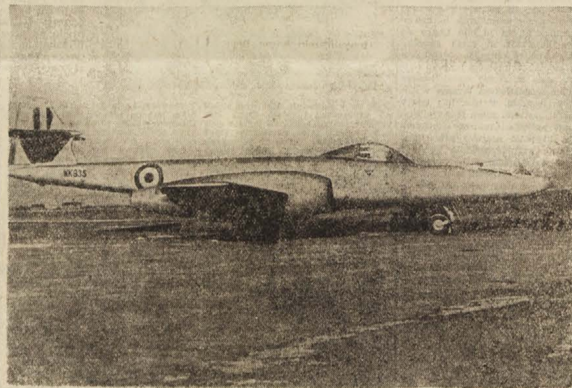
Prvo letalo na reaktivni pogon, izdelano v tovarni Armstrong Whitworth v Veliki Britaniji. V njem pilot med poletom leži, in sicer zadaj ali spredaj. Pilotiranje leže pride v poštev pri posebno hitrem poletu. Če pilot v letalu leži, je namreč vpliv hitrosti na obtok njegove krvi manjši.
